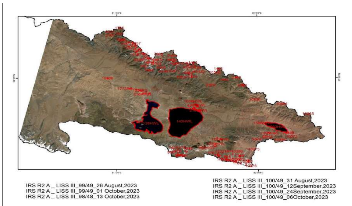
Fig. 7.4 (d): IRS-R2, LISS III, 99/49 & 100/49
